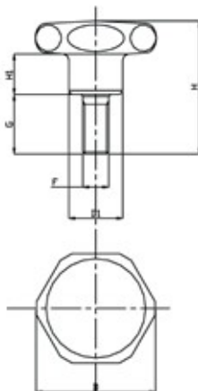
VOLANINI INOX A LOBI - FILETTO MASCHIO STAINLESS STEEL KNOBS - MALE
